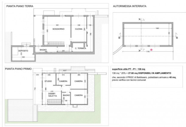
PLANIMETRIA INDICATIVA
