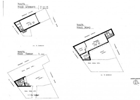
PIANIMETRIA INDICATIVA
