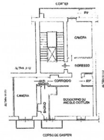
PIANTA PIANO SECONDO (111 f t) H media: 3,30 m
