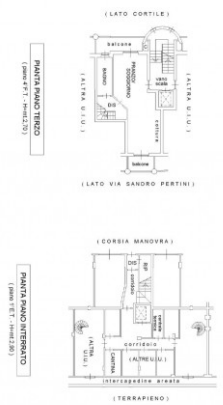
PLANIMETRIA INDICATIVA
