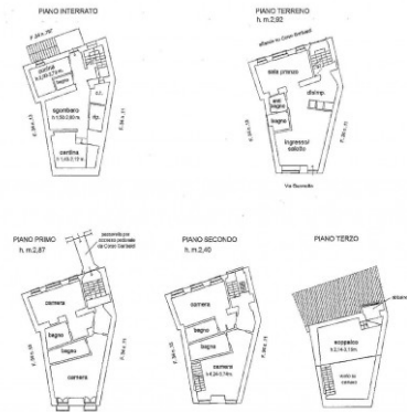
PLANIMETRIA INDICATIVA
