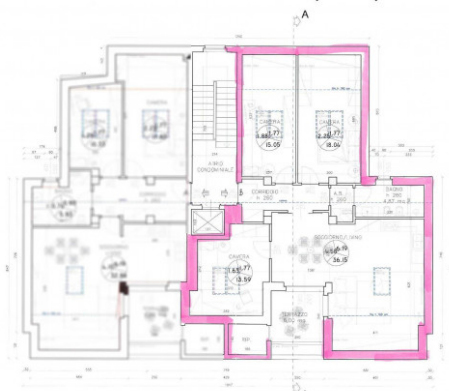
PLANIMETRIA INDICATIVA
