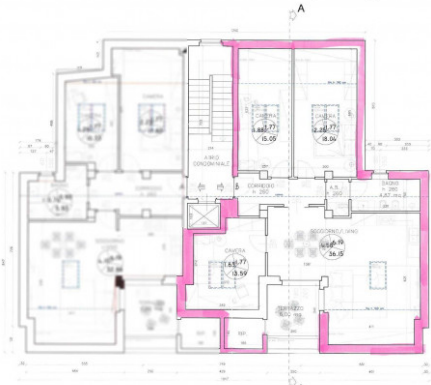
PLANIMETRIA INDICATIVA
