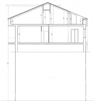
PLANIMETRIA INDICATIVA
