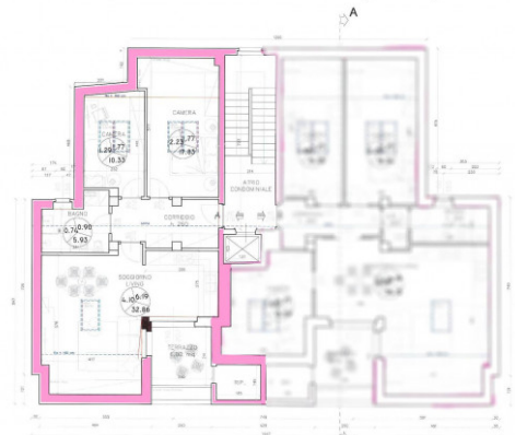
PLANIMETRIA INDICATIVA
