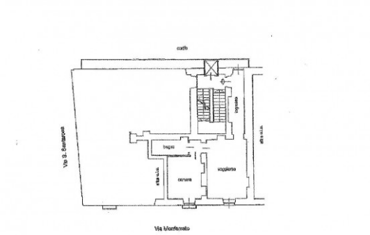
PIANTA PIANO TERZO (4° f.t.) H md. 2.70
