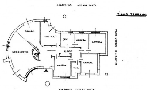
PLANIMETRIA INDICATIVA
