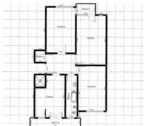
PLANIMETRIA INDICATIVA
