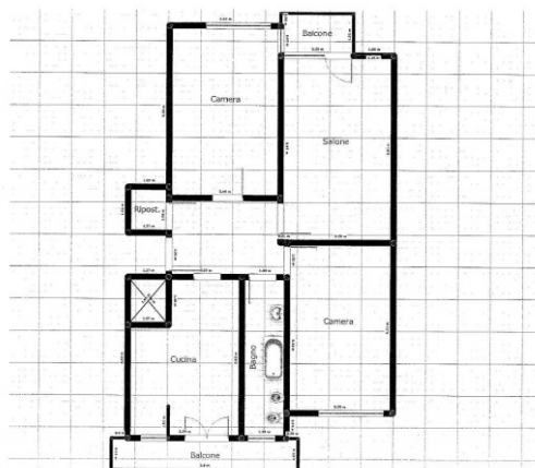
PLANIMETRIA INDICATIVA
