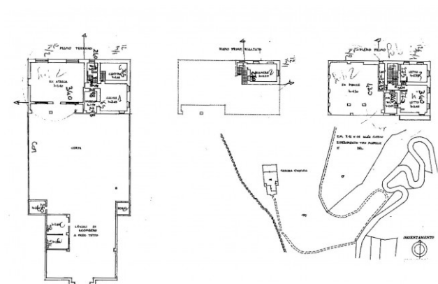
PLANIMETRIA INDICATIVA
