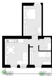
APPARTAMENTO G - piano primo scala 1:50
