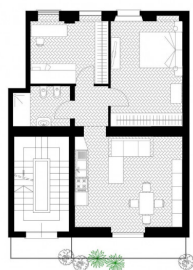
APPARTAMENTO I - piano primo scala 1:50
