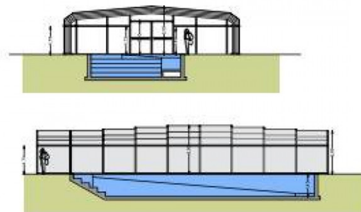
SEZ. LONGITUDINALE
