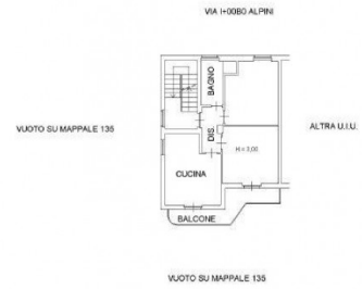
PIANO PRIMO
