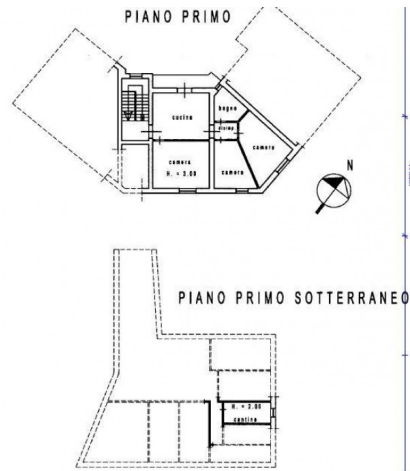
PIANO PRIMO
