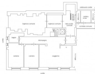
PLANIMETRIA INDICATIVA
