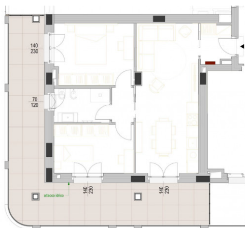
PLANIMETRIA INDICATIVA
