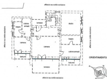
PIANTA PIANO PRIMO - H. 3.00 mt PLANIMETRIA INDICATIVA
