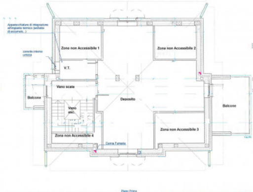
PLANIMETRIA INDICATIVA
